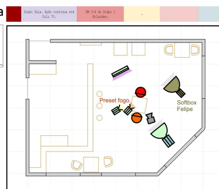
Planta baixa Cena 008 Plano 034
