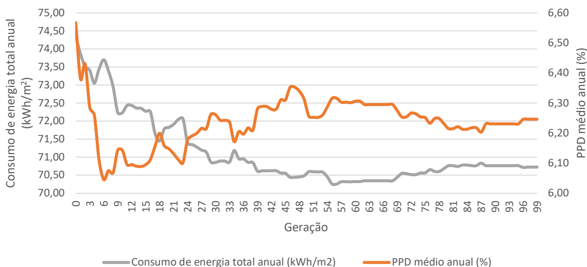
Figura 22. Valores médios das funções objetivo consumo de energia anual e PPD médio anual por geração
