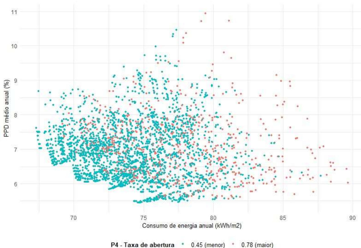
Figura 30 - Funções objetivo com todas soluções diferenciadas pelas opções da variável de projeto P4 taxa de abertura
