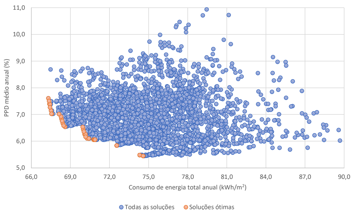
Figura 23. Funções objetivo com todas soluções simuladas na otimização multiobjetivo
