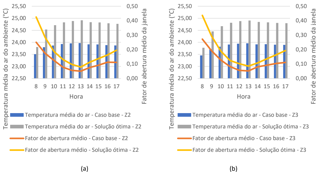
Figura 38 – Valor médio horário da temperatura média do ambiente e do fator de abertura médios da janela dos ambientes Z2 da fachada leste (a) e Z3 da fachada oeste (b)
