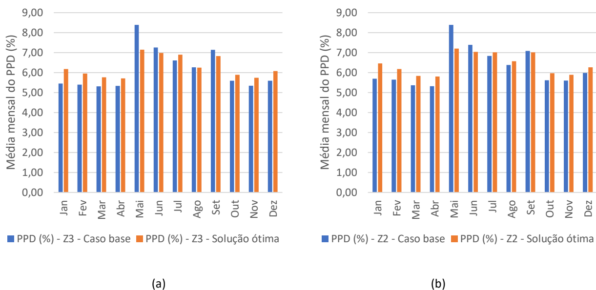
Figura 39 – Valor médio horário de PPD nas horas de ocupação dos ambientes Z2 da fachada leste (a) e Z3 da fachada oeste (b)
