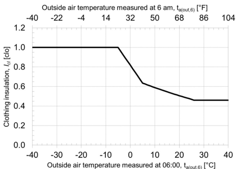
Figura 12. Variação do isolamento do vestuário em função da temperatura externa
