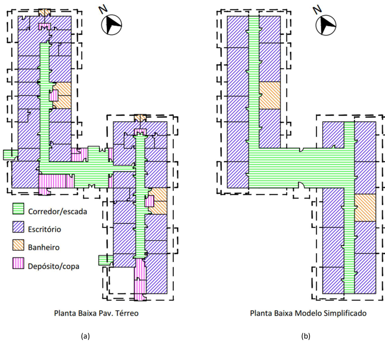
Figura 9. Planta baixa do pavimento térreo (a) e planta baixa do modelo simplificado para simulação (b)
