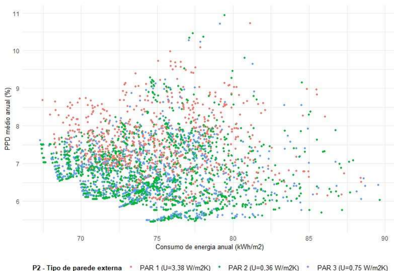
Figura 28 - Funções objetivo com todas soluções diferenciadas pelas opções da variável de projeto P2 tipo de parede externa
