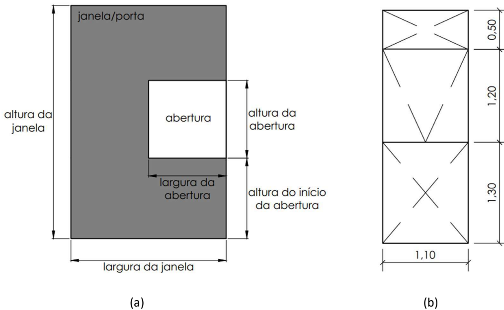
Figura 15. Frações de aberturas consideradas para o cálculo dos fatores (a) e geometria da janela de escritório considerada para os cálculos dos fatores (b)
