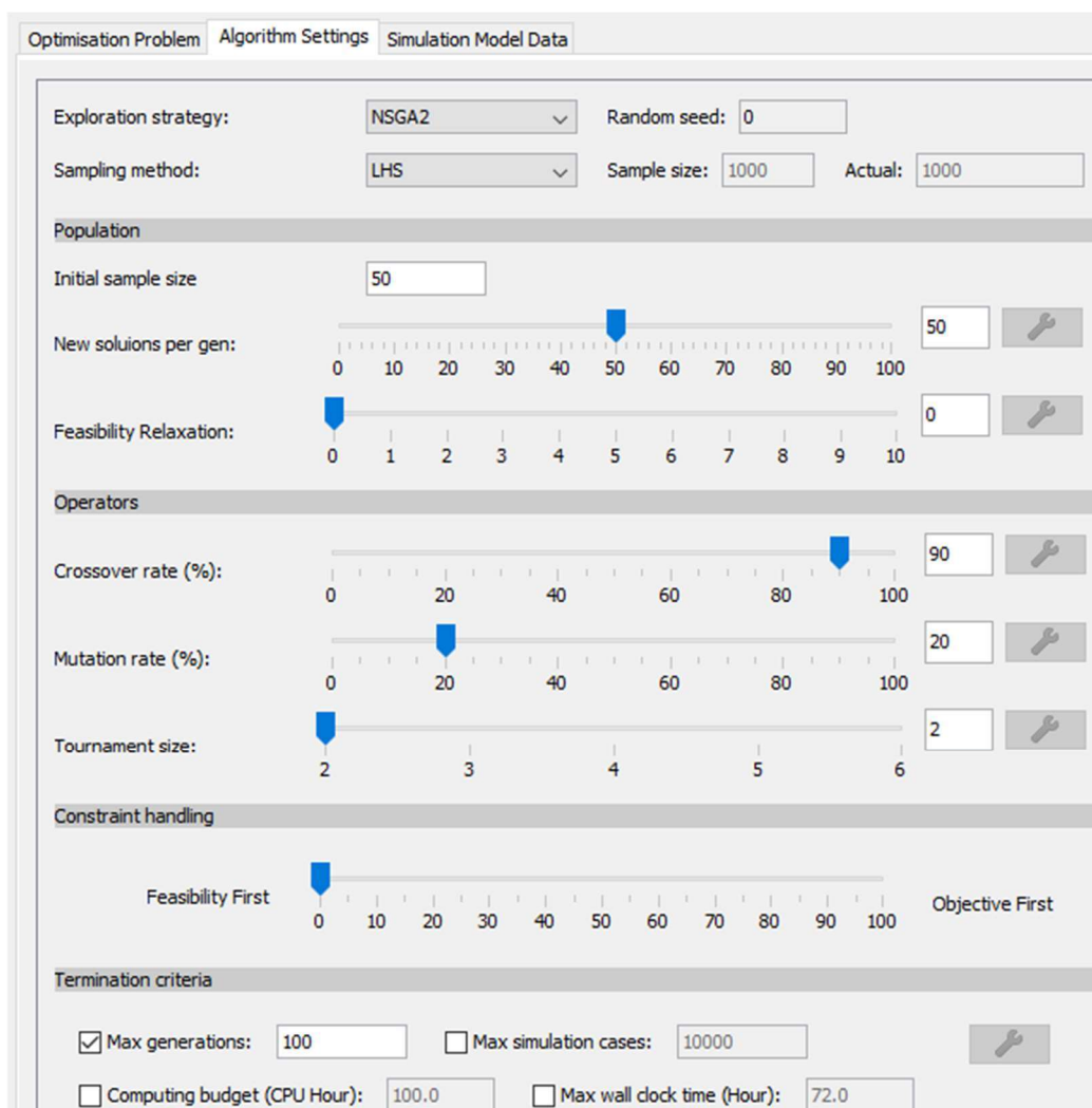
Figura 19. Interface da configuração dos parâmetros do algoritmo NSGA-II no programa jEPlus+EA
