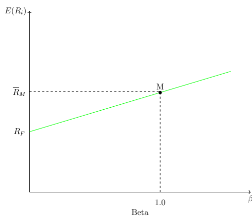
Figura 1.8: Relação Retorno-Beta
