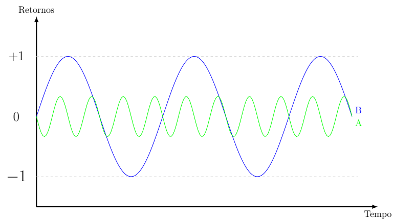
Figura 1.3: Correlação nula = 0
