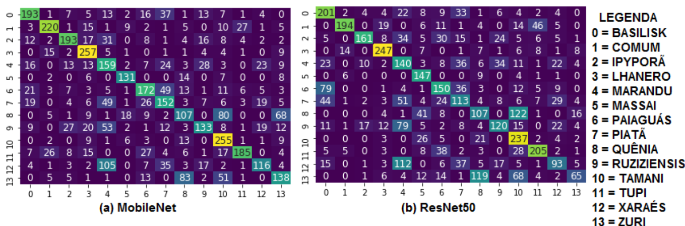
Figura 5.28: Área Geral período de seca - classificação por Cultivar matriz confusão MobileNet e ResNet50
