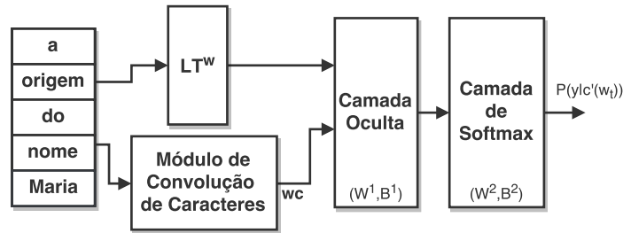
Figura 2.6: Rede proposta por CharWNN.
