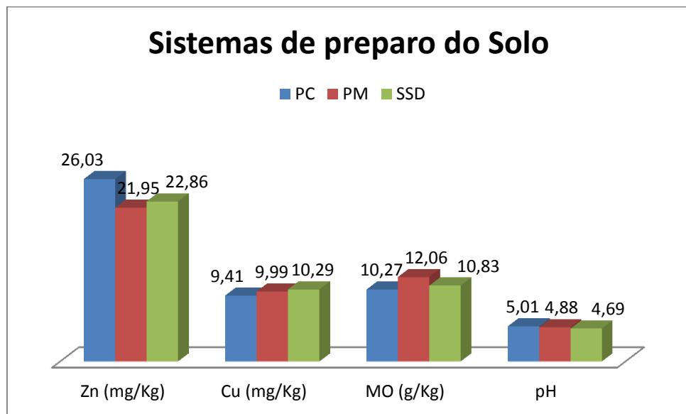
Figura 1- Concentrações médias de Zn, Cu, MO e pH em Latossolo Vermelho distrófico de área submetida aos diferentes preparos dos solos (Janeiro de 2013).
