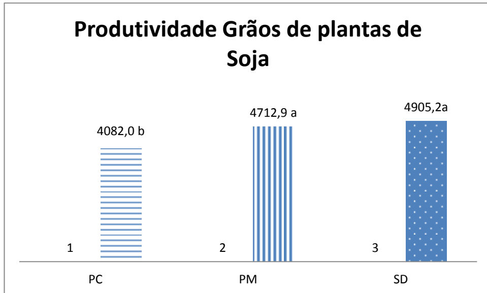
Gráfico 2- Produtividade da soja- safra 2012/2013, área experimental UFMS/CPCS. Foi aplicado o Teste de Scott-Knott ao nível de 5% de probabilidade, CV = 8,18 %.
