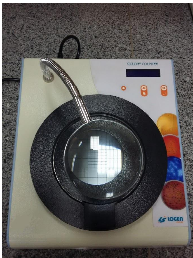
Figura 6: Contador de colônias eletrônico/digital utilizado na pesquisa
