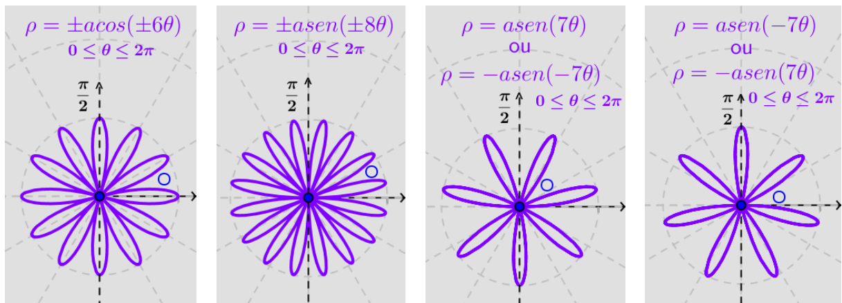
Figura 37 - Rosácea de |n| pétalas, com n \in \mathbb{Z}
