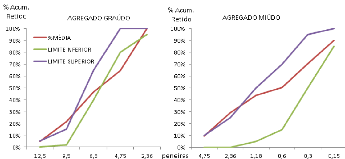
Figura 28. Curva granulométrica do RCD Fonte: Elaborado pelo autor
