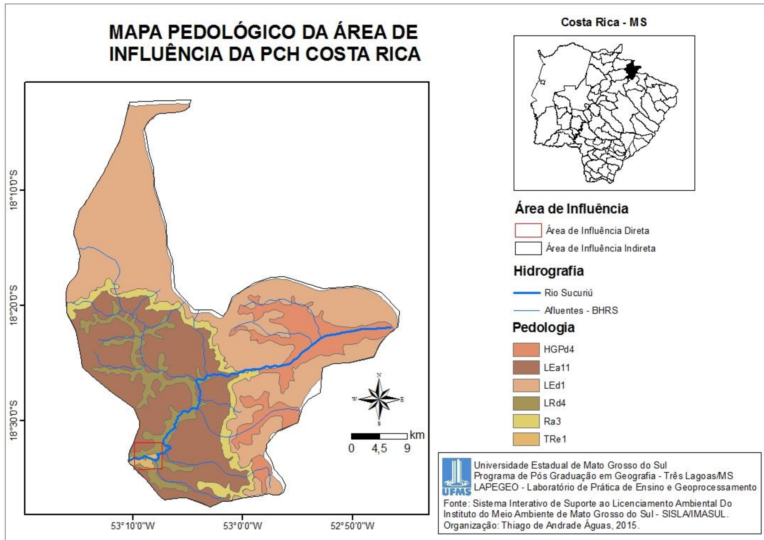
Figura 14 - Mapa pedológico da Área de Influência da PCH Costa Rica. Organização: Thiago de Andrade Águas, 2015.
