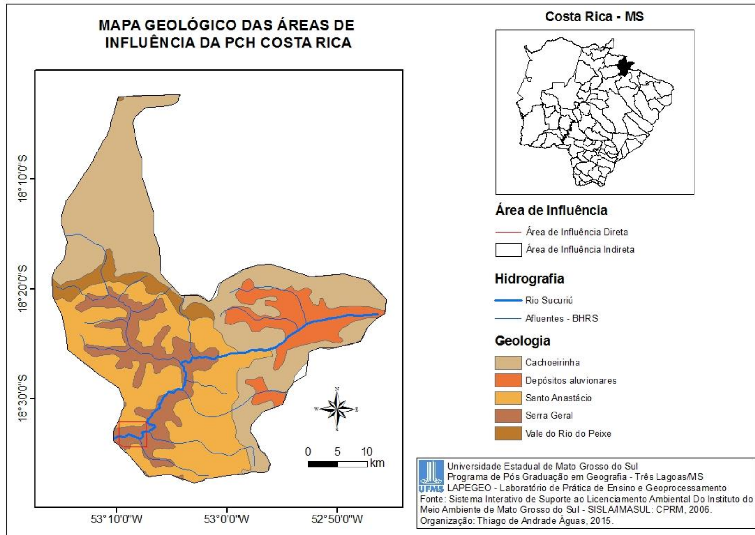
Figura 13 – Mapa geológico das áreas de influência da PCH Costa Rica. Organização: Thiago de Andrade Águas, 2015.
