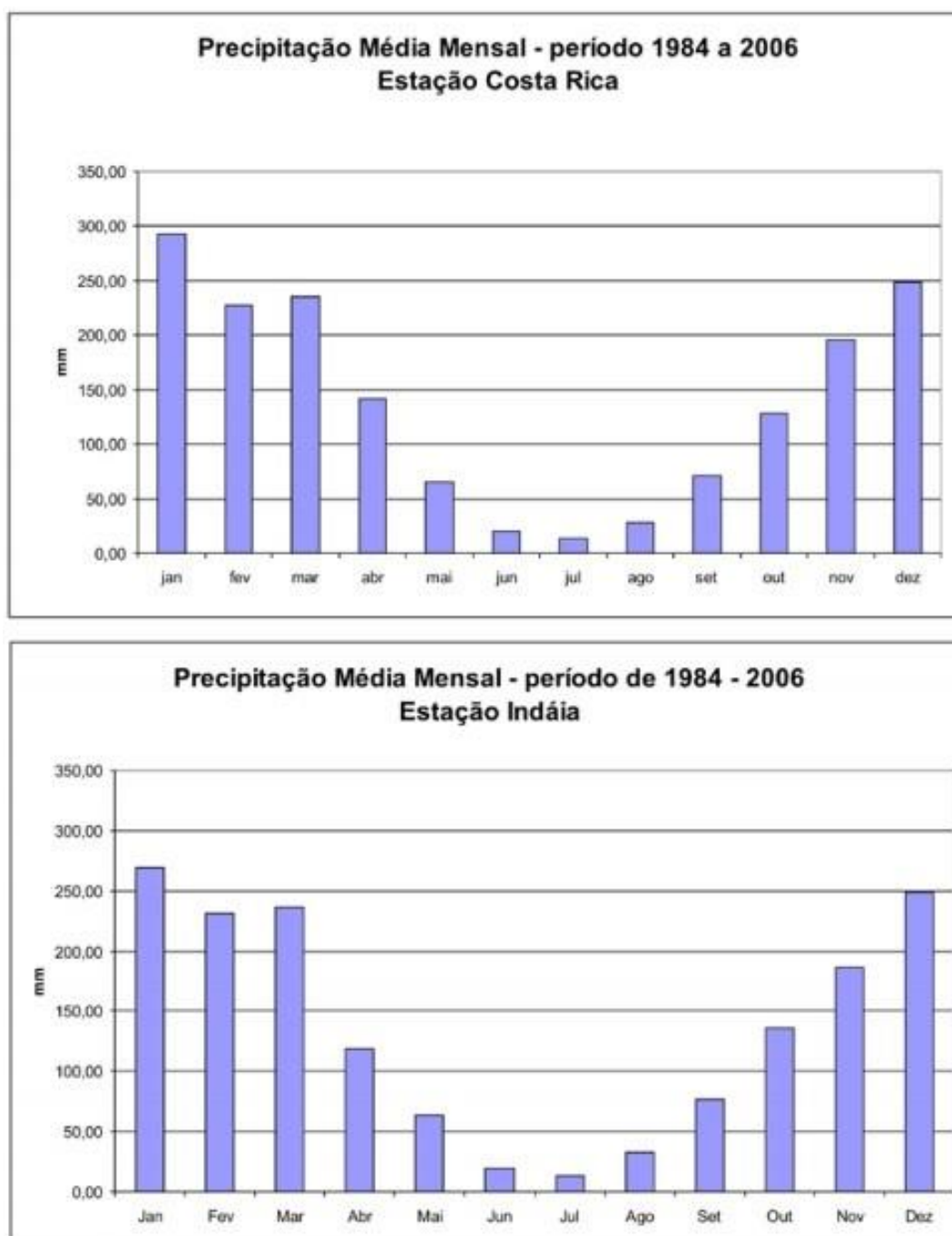
Gráfico 2 - Médias mensais das estações localizadas no alto curso da BHRS. Fonte: Ferreira, 2011 (adaptado).
