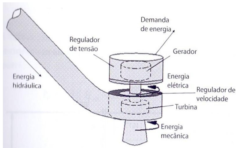
Figura 2 – Processo de conversão de energia. Fonte: Flórez, 2012.
