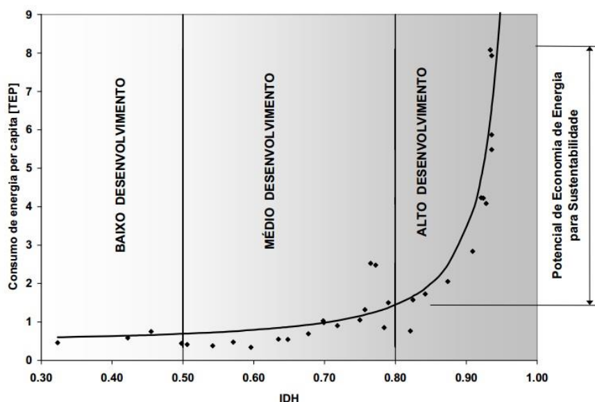
Gráfico 1 – Consumo de Energia per capta em TEP/ano versus IDH.
