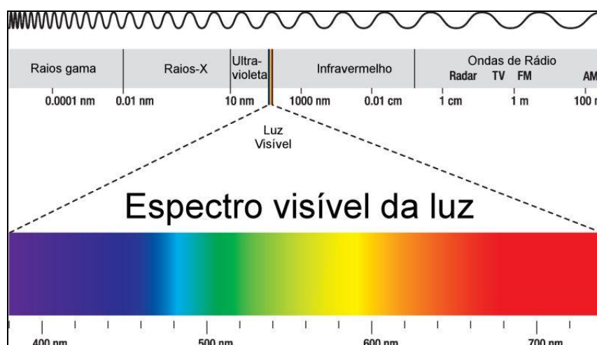
Figura 3 - Espectro eletromagnético.
