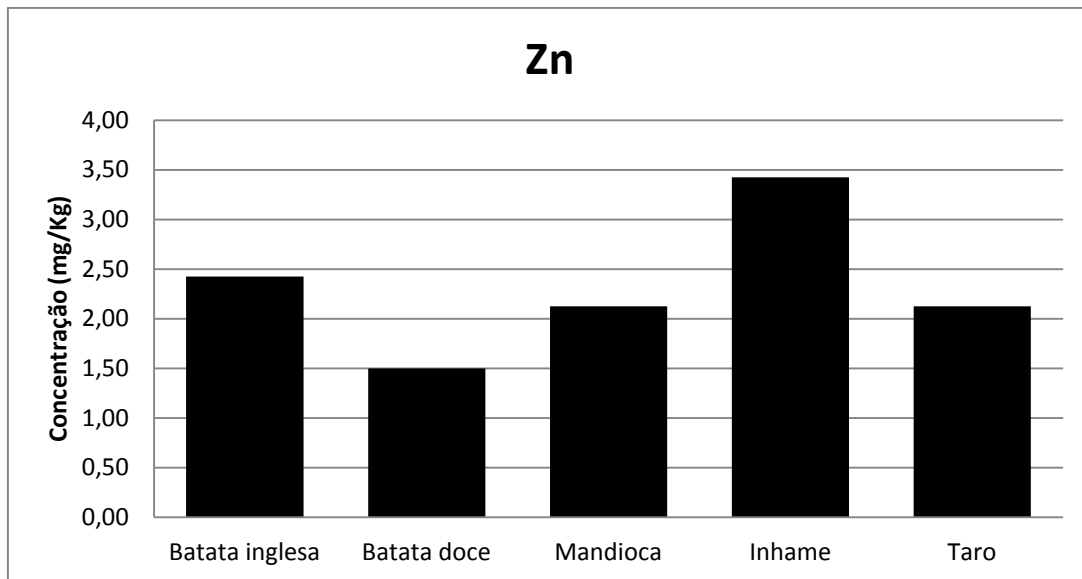
Figura 2 - Gráfico representando a comparação das concentrações (mg/kg) de zinco na amostra úmida em tubérculos estudados.
