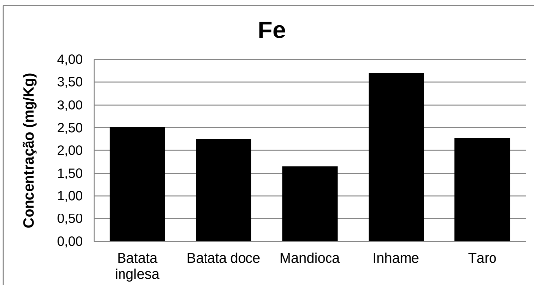
Figura 4 - Gráfico representando a comparação das concentrações (mg/kg) de ferro na amostra úmida em tubérculos estudados.
