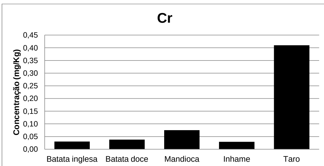
Figura 7 - Gráfico representando a comparação das concentrações (mg/kg) de cromo na amostra úmida em tubérculos estudados.
