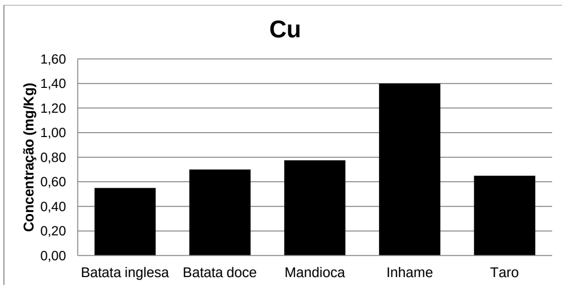
Figura 3 - Gráfico representando a comparação das concentrações (mg/kg) de cobre na amostra úmida em tubérculos estudados.
