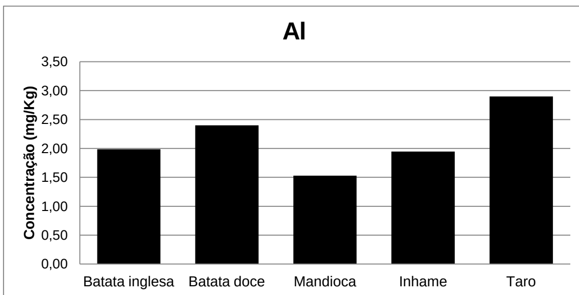
Figura 6 - Gráfico representando a comparação das concentrações (mg/kg) de alumínio na amostra úmida em tubérculos estudados.
