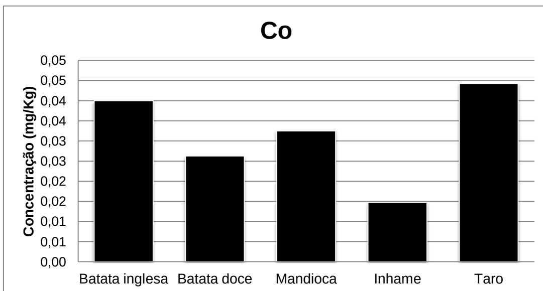
Figura 10 - Gráfico representando a comparação das concentrações (mg/kg) de cobalto na amostra úmida em tubérculos estudados.
