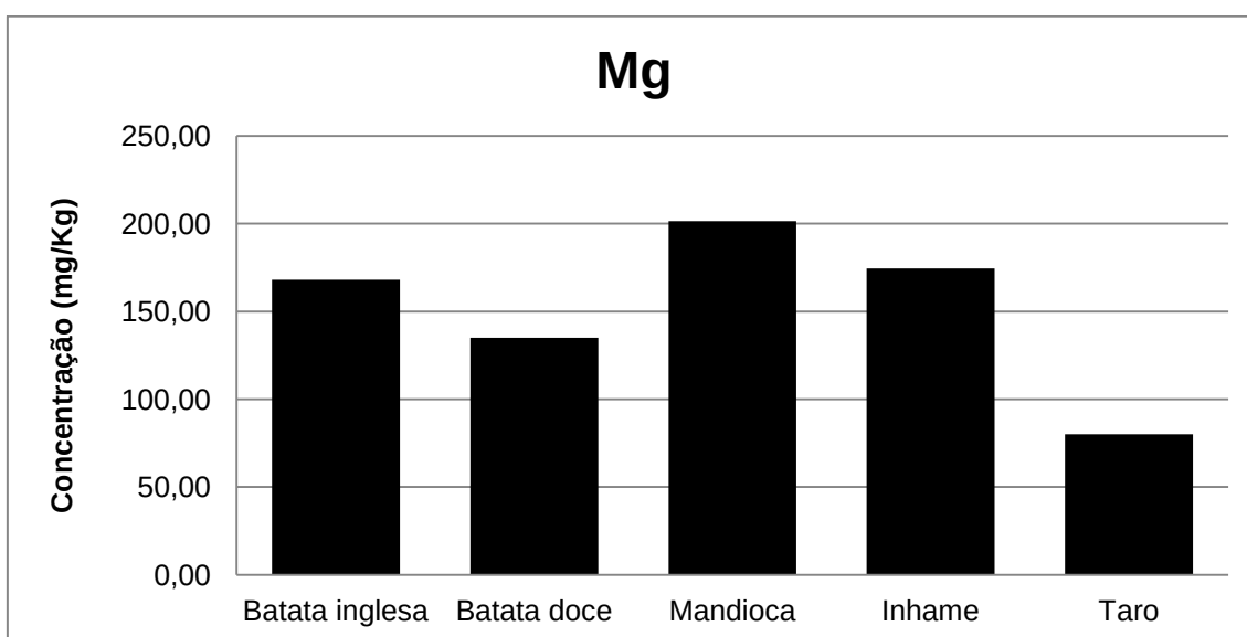
Figura 1 - Gráfico representando a comparação das concentrações (mg/kg) de magnésio na amostra úmida em tubérculos estudados.
