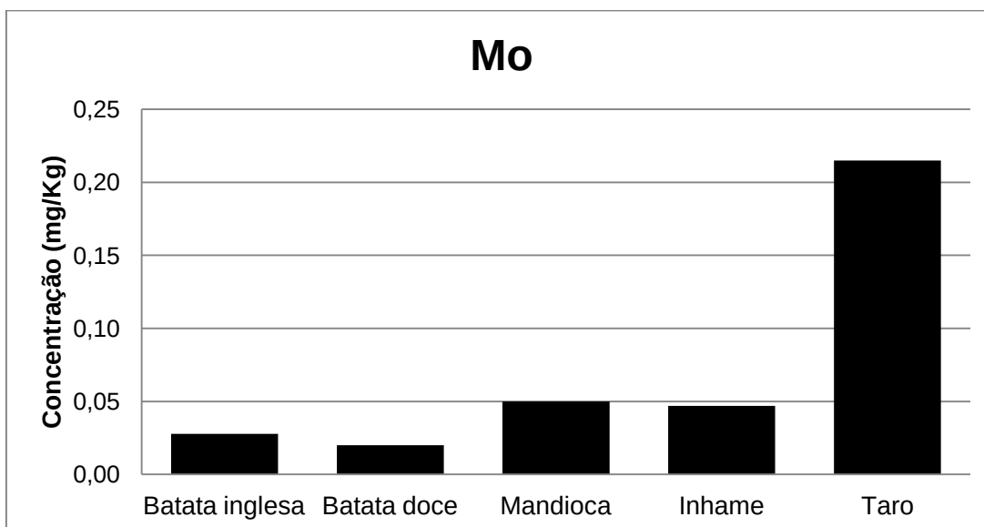
Figura 11 - Gráfico representando a comparação das concentrações (mg/kg) de molibdênio na amostra úmida em tubérculos estudados.
