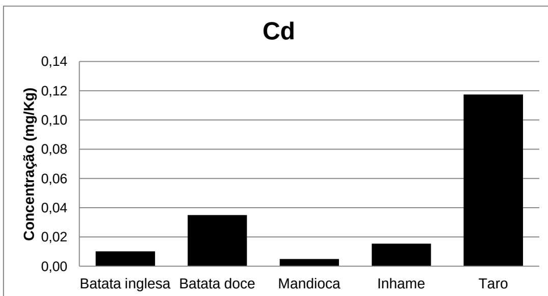
Figura 8 - Gráfico representando a comparação das concentrações (mg/kg) de cádmio na amostra úmida em tubérculos estudados.
