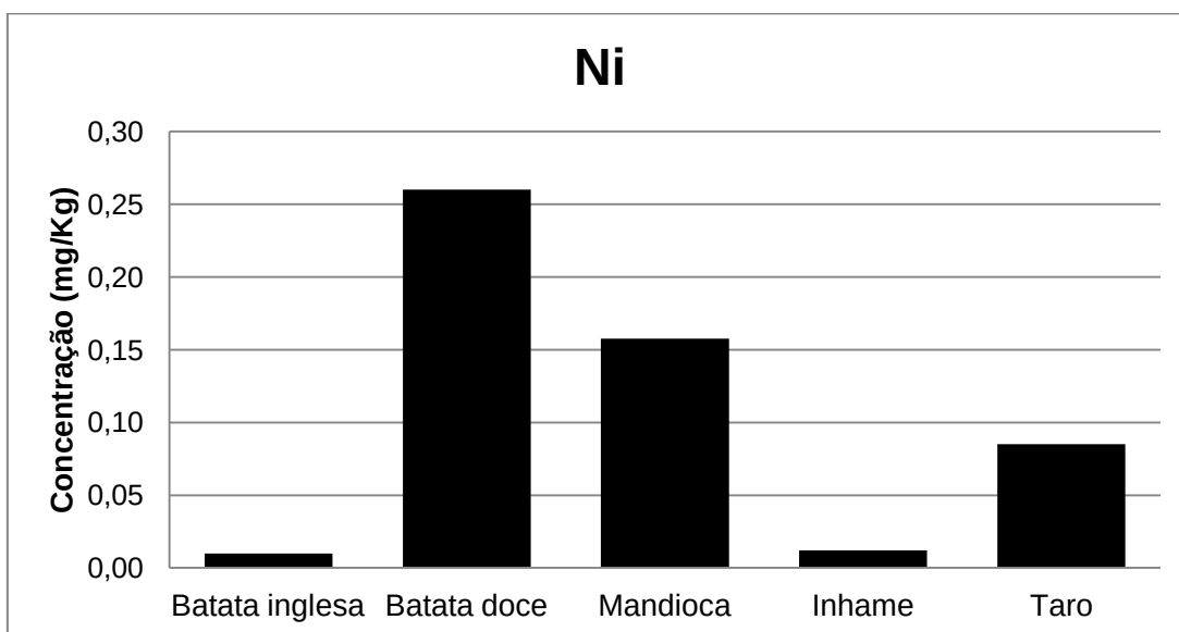
Figura 9 - Gráfico representando a comparação das concentrações (mg/kg) de níquel na amostra úmida em tubérculos estudados.
