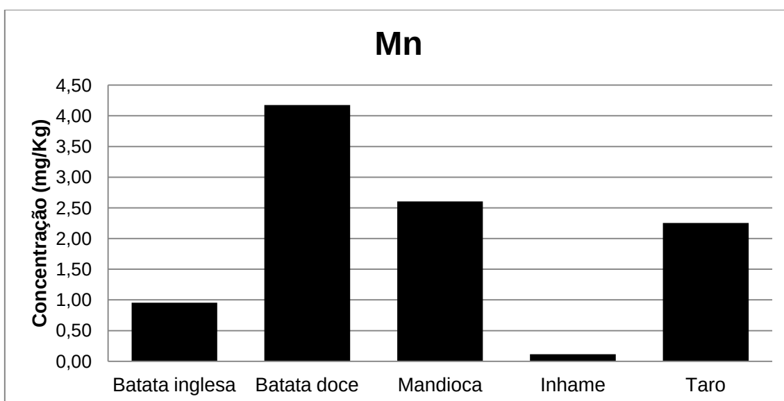
Figura 5 - Gráfico representando a comparação das concentrações (mg/kg) de manganês na amostra úmida em tubérculos estudados.
