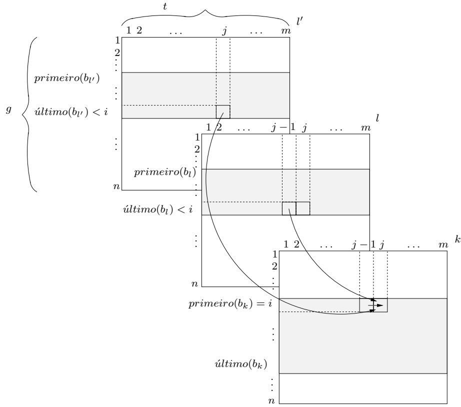
Figura 3.3: Matrizes bidimensionais representando os blocos b_{l'} , b_l e b_k em S , necessárias para preenchimento da posição S[i][j][k] quando i = \text{primeiro}(b_k) . As setas indicam as posições anteriormente preenchidas que serão consultadas para o cálculo do valor de S[i][j][k] e as áreas sombreadas esboçam as regiões utilizadas em S para representar os blocos b_{l'} , b_l e b_k (figura adaptada de Kishi e Adi [24, 25]).
