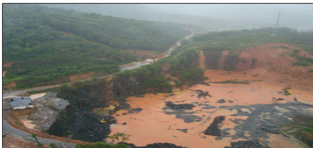
Figura 4: Movimentação de Massa e Quebra de Barreira, na BR 101-SC, entre Jaraguá do Sul e Massaranduba, no verão de 2008 Fonte: WAG CBJR (Dez., 2008)
