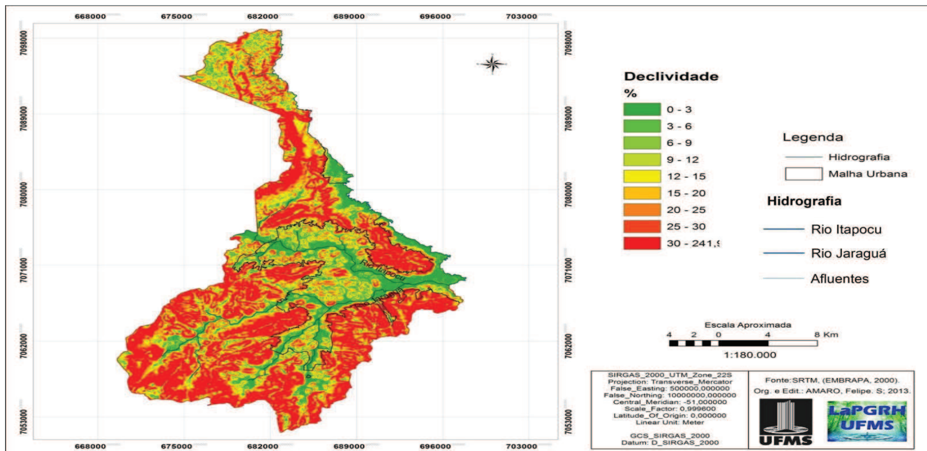
Figura 9: Mapa da declividade do Município de Jaraguá do Sul – SC. Fonte: Dados altimétricos da imagem SRTM.
