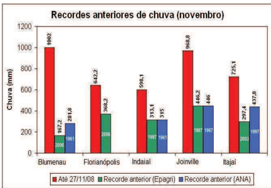
Figura 6: Recordes de novembro e respectivos anos de ocorrência, nas estações da Epagri e ANA, na primavera de 2008. Fonte: Epagri 2008.
