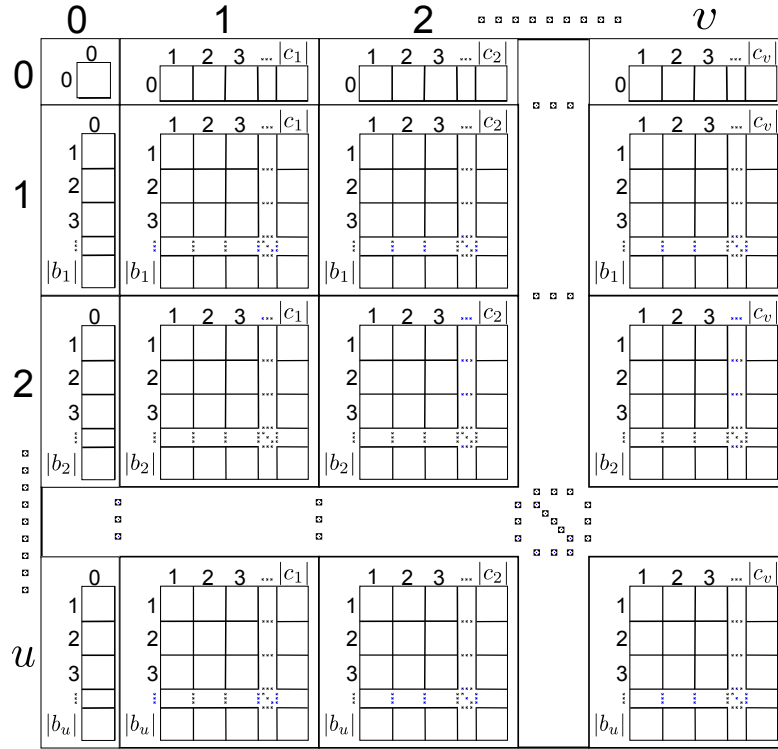
Figura 4.1: Representação da matriz de alinhamento de segmentos quadridimensional M utilizando uma combinação de submatrizes de alinhamento bidimensionais.
