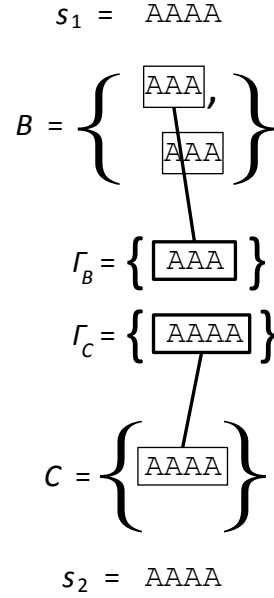
Figura 3.5: Uma instância que mostra que a Recorrência 3.3 não resolve o PASG.
