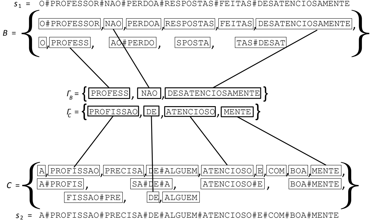
Figura 3.1: Uma instância do PASG.
