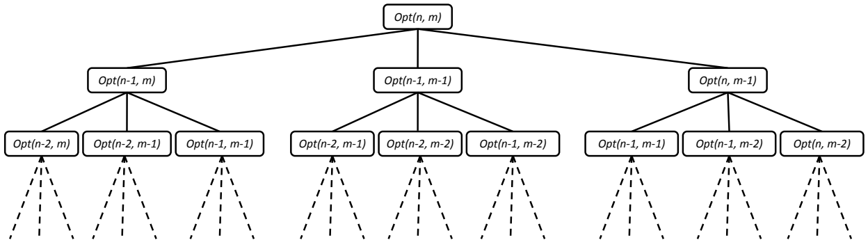
Figura 2.3: Árvore de recursão para Opt(n, m) .
