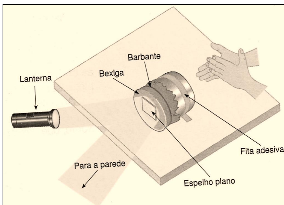
Figura 6- Material proposto para visualizar ondas sonoras (PENTEADO e TORRES, 2005, p. 128).
