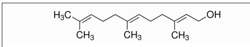
Figura 4 - Estrutura química do tt-farnesol (C 15 H 26 O).
