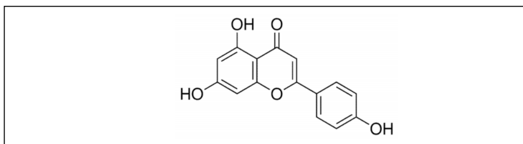
Figura 3 - Estrutura química da apigenina ( C_{15}H_{10}O_5 ).
