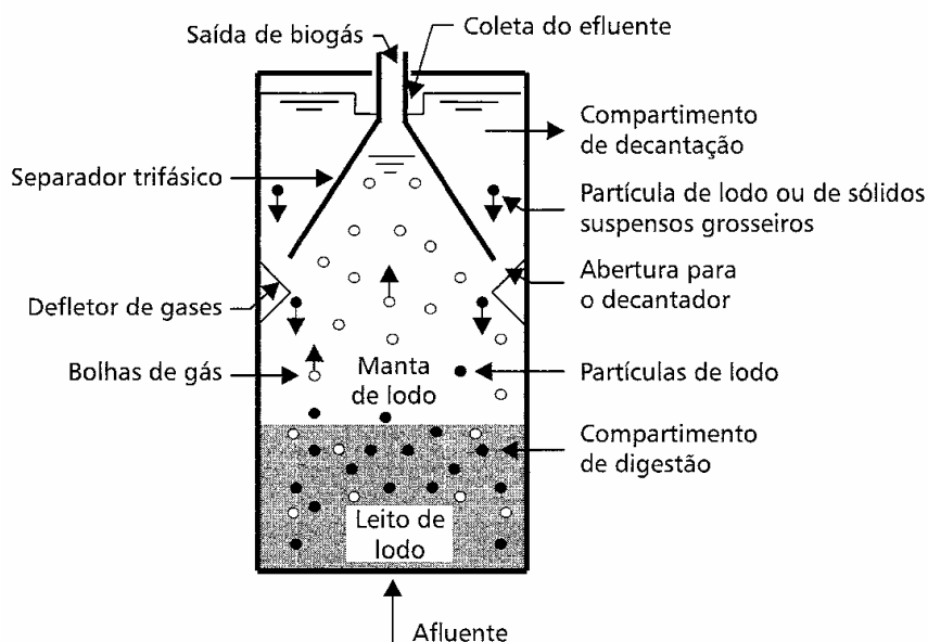
FIGURA 3.7 - Estrutura básica de um reator UASB. Fonte: Chernicharo (1997).
