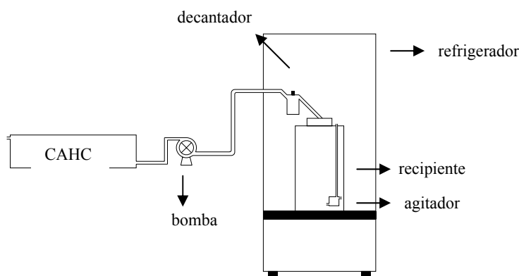
FIGURA 4.3. Esquema do sistema de abastecimento da CAHC.
