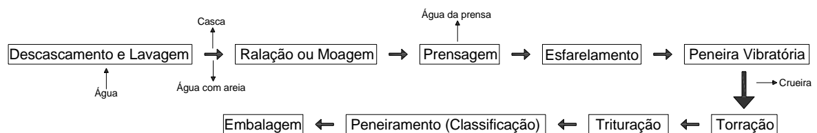
FIGURA 3.2 - Fluxograma geral de uma farinheira. Fonte: Adaptado de Cereda & Vilpoux (2003).
