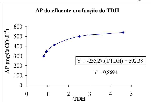
FIGURA 6.2 - Ajuste dos dados de AP em função do TDH.
