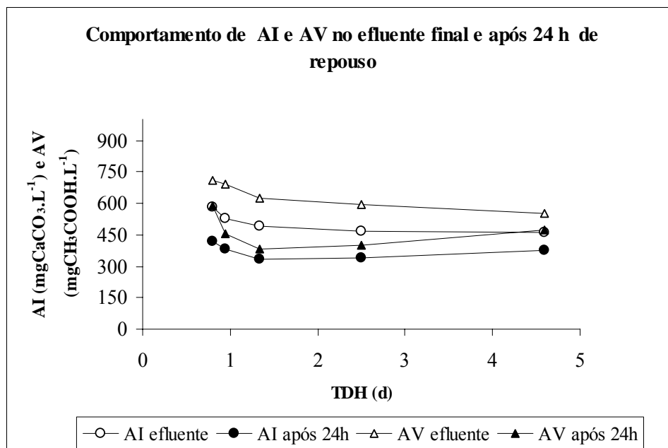
FIGURA 5.4 - Comportamento da AI e da AV após 24 h de repouso.
