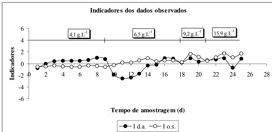
FIGURA 6.5 - Comportamento dos dados observados nas fases III, IV, V e VI expressos através dos indicadores de tratabilidade do sistema.
