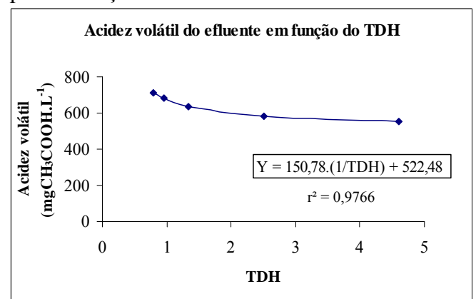
FIGURA 6.3 - Ajuste dos dados de AV em função do TDH.
