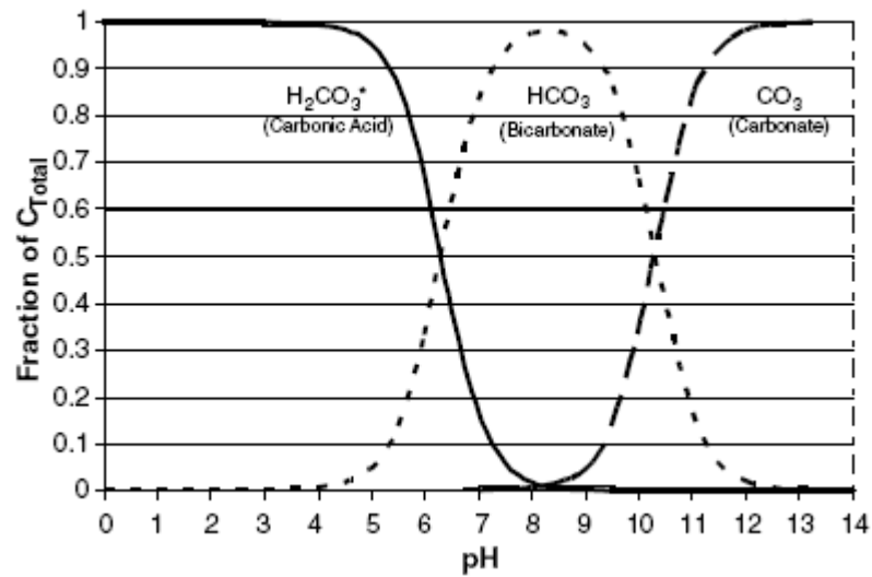
FIGURA 3.9 - Solubilidade e especiação do CO 2 em função do pH. Fonte: Snoeyink & Jenkins (1980) citado por Taconi et al. (2007).
