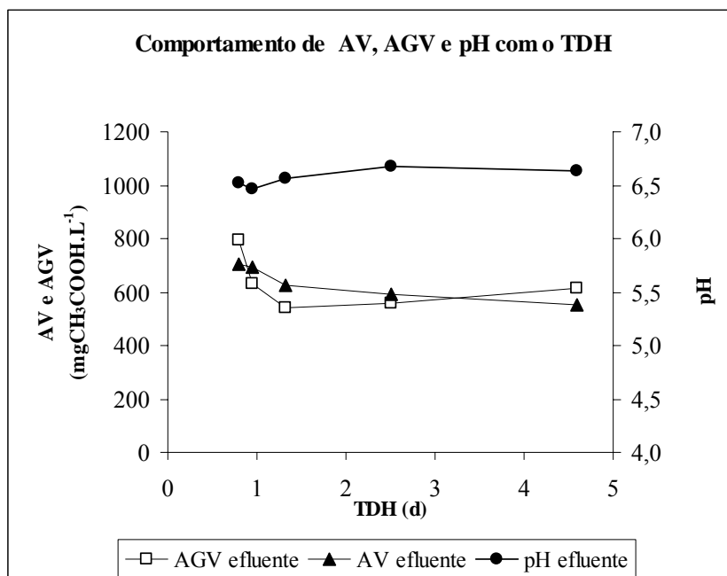
FIGURA 5.2 - Comportamento dos parâmetros AGV, AV e pH no efluente da CAHC nos TDH testados.
