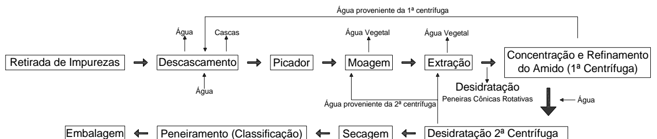
FIGURA 3.1 - Fluxograma geral do processo produtivo de fecularias. Fonte: Adaptado de Vilpoux (2003).
