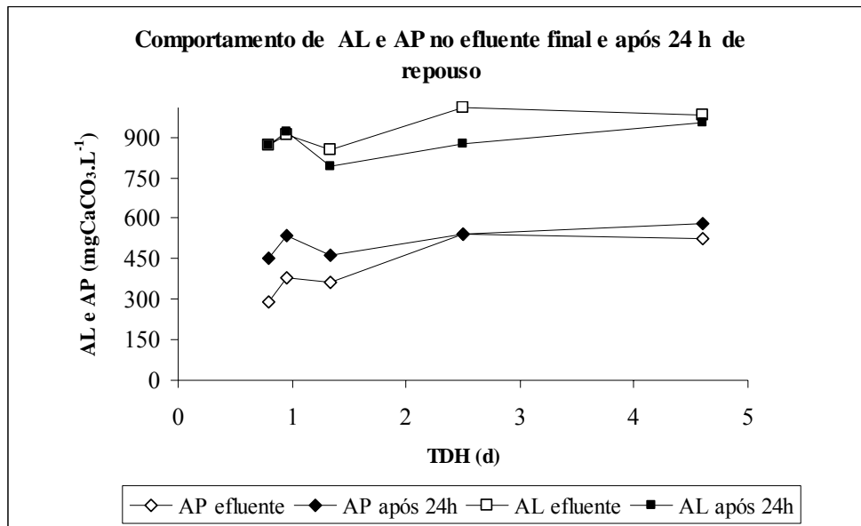
FIGURA 5.3 - Comportamento do efluente da CAHC na saída e após 24 h de repouso, quanto à alcalinidade total e parcial (bicarbonato).
