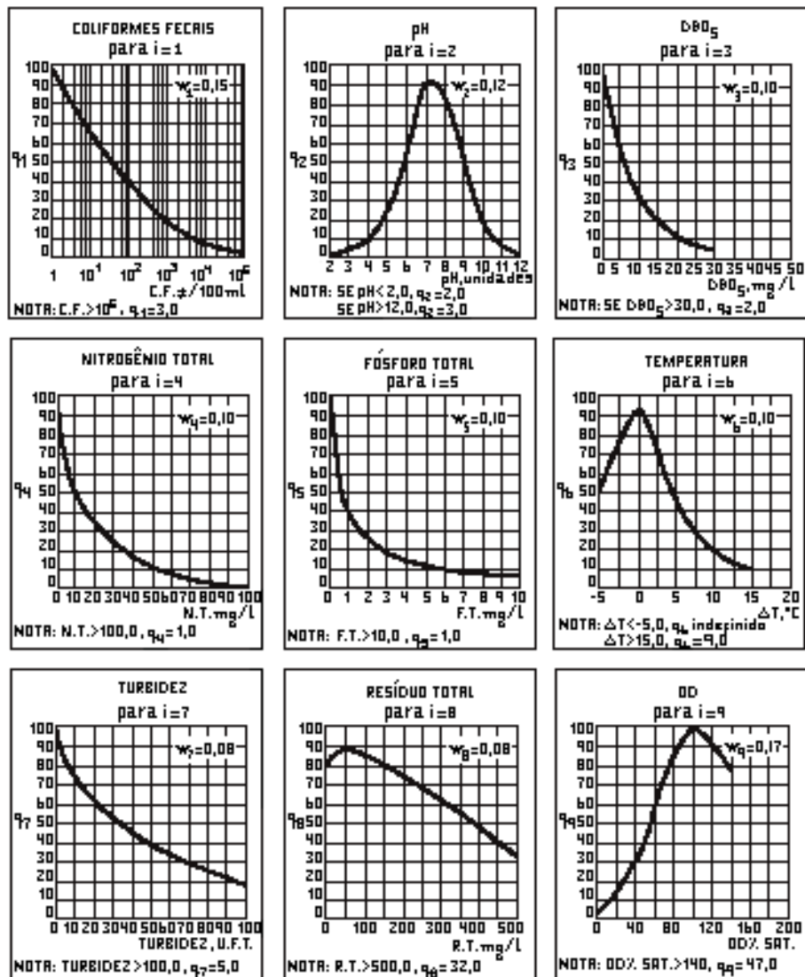
Figura 3.1 - Curvas de variação dos parâmetros IQA_{Cetesb} .
