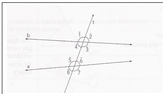
Figura 19- Ângulos de retas com uma transversal (IEZZI; DOLCE; MACHADO, 2005, p. 89).
