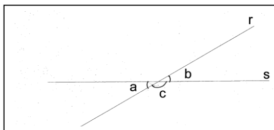
Figura 1–Demonstração da congruência de ângulos opostos pelo vértice (1).
