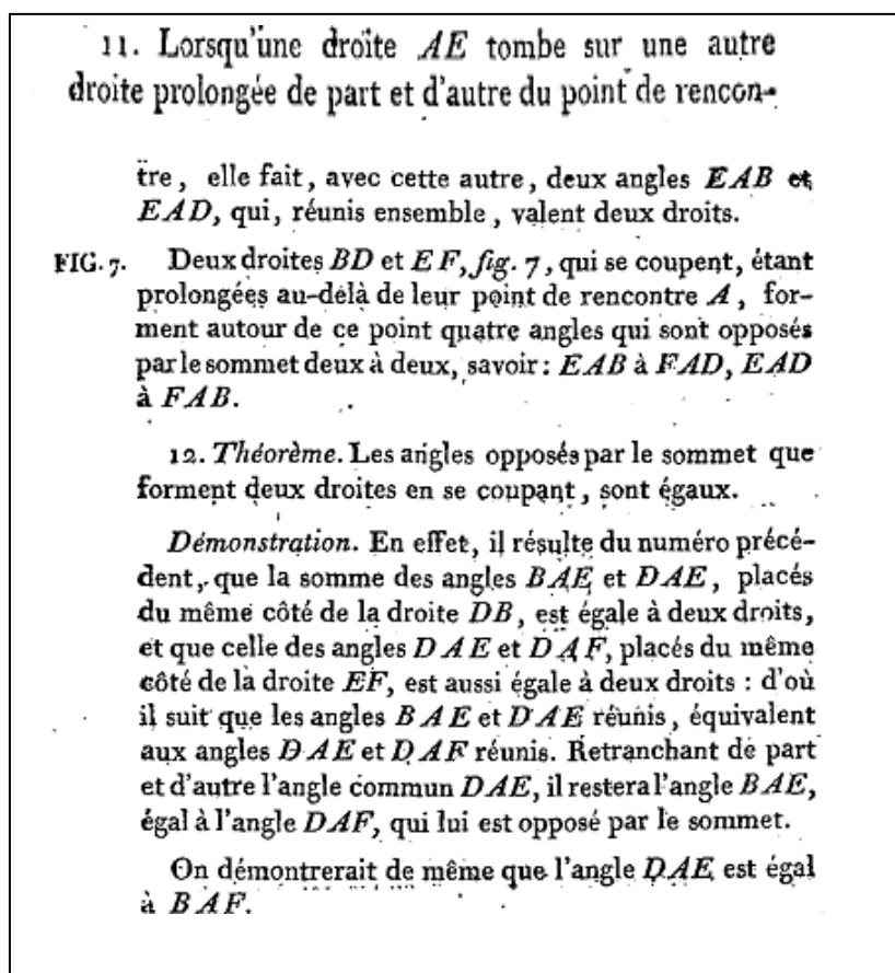
Figura 26 – Proposição de (LACROIX, 1808, p. 7-8)
