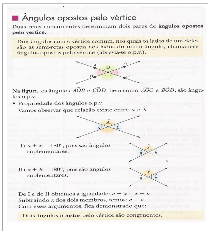
Figura 9 –O.P.V.(1) (BARROSO, 2006, p. 77)
