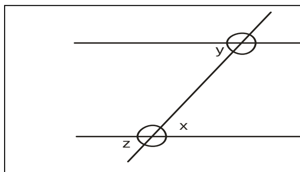
Figura 8—Retas paralelas cortadas por uma transversal
