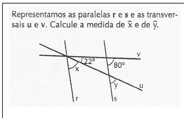
Figura 24-Ângulos formados por paralelas (3) (CENTURIÓN; JAKUBOVIC; LELLIS, 2008, p. 145)
