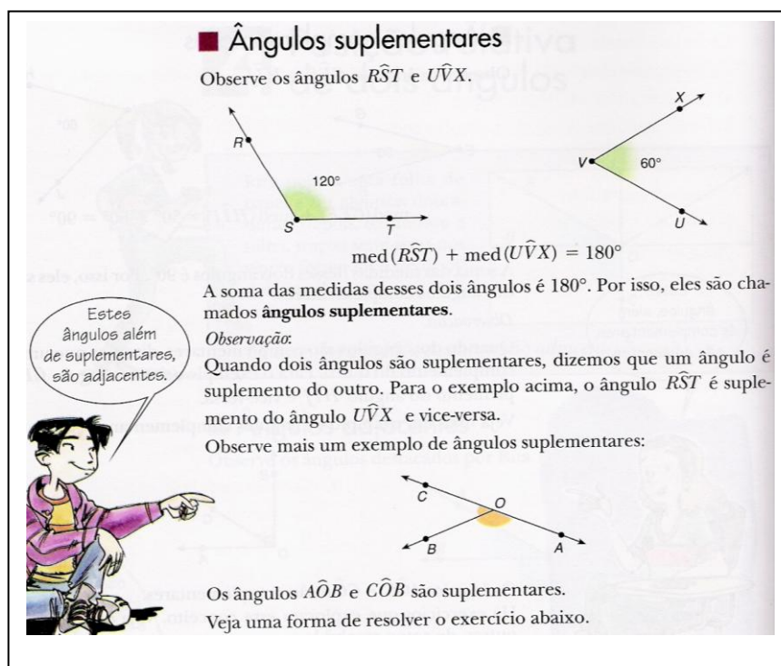
Figura 12-Ângulos suplementares ( BARROSO, 2006, p. 60).
