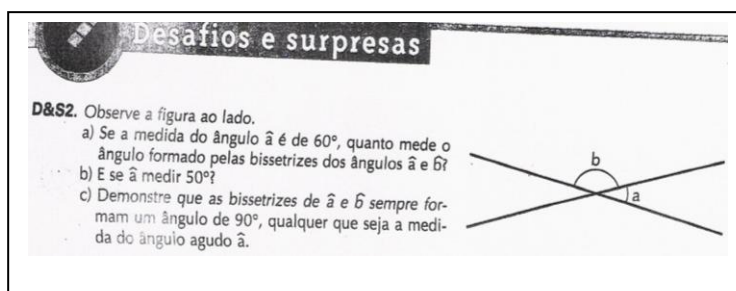
Figura 21-Atividade para demonstrar (CENTURIÓN; JAKUBOVIC; LELLIS, 2008, p. 141)
