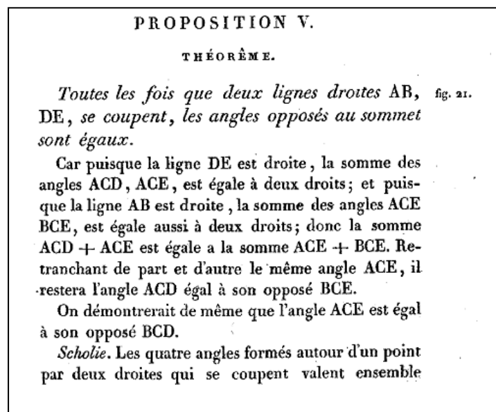
Figura 28—Proposição V de Legendre (LEGENDRE, 1817 p. 9-10)
