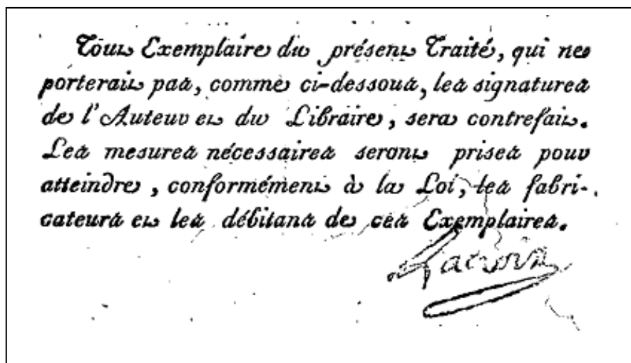
Figura 25- Advertência (LACROIX, 1808, p. s/n )
