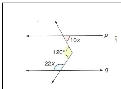
Figura 10–Ângulos entre paralelas (BARROSO, 2006, p. 83)
