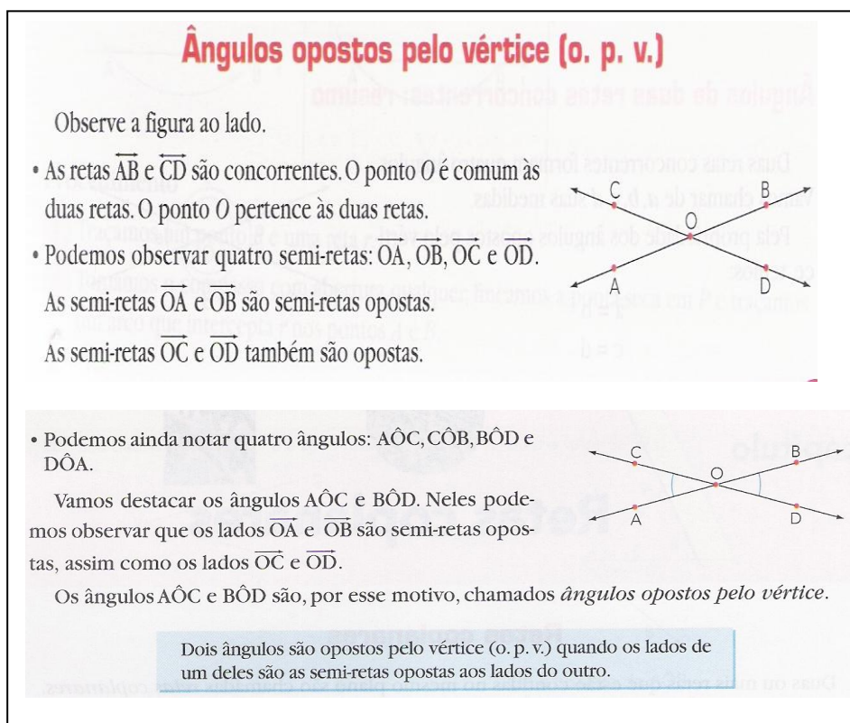
Figura 18-Ângulos o.p.v. (1) (IEZZI; DOLCE; MACHADO, 2005, p. 85-86).
