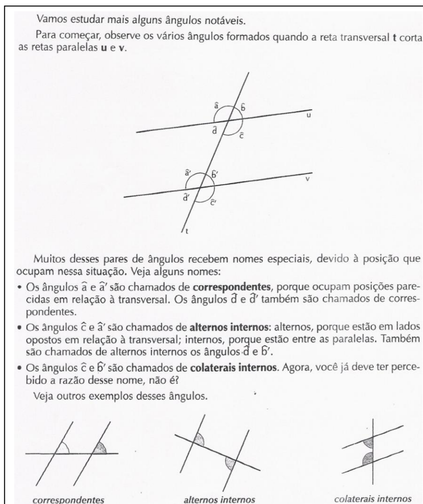
Figura 22-Ângulos formados por paralelas e transversais (1) (CENTURIÓN; JAKUBOVIC; LELLIS, 2008, p. 142)
